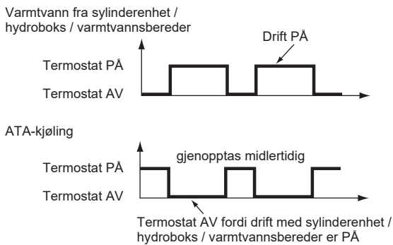
Driftsstatus når ATA-kjøling og varmtvannstilførsel skal kjøres samtidig
