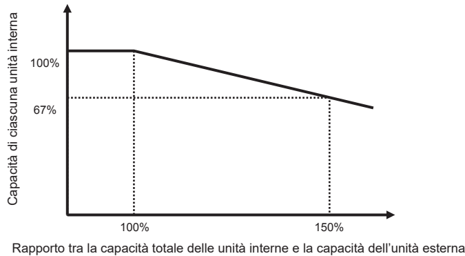
Funzionamento quando la capacità totale delle unità interne in funzione supera la capacità dell'unità esterna.
