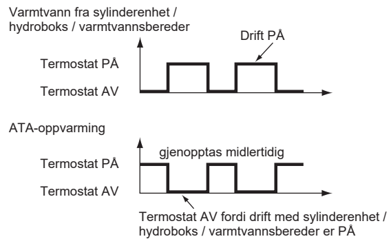
Driftsstatus når ATA-oppvarming og varmtvannstilførsel skal kjøres samtidig
