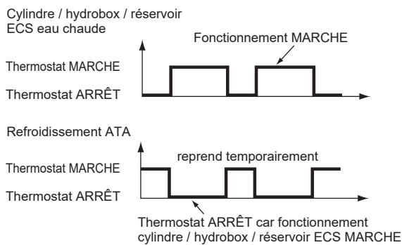
État de fonctionnement lorsque les modes Refroidissement ATA et alimentation en eau chaude sont utilisés en même temps
