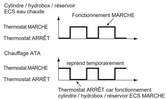
État de fonctionnement lorsque les modes Chauffage ATA et alimentation en eau chaude sont utilisés en même temps
